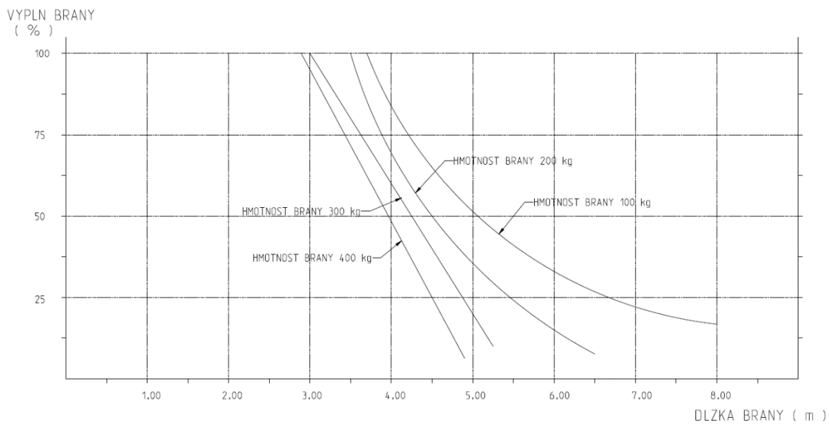
VZTAH PERCENTA VYPLNE BRANY VYSKY 2 200 mm OD JEJ DLZKY HMOTNOST JE ROVNOMERNE ROZLOZENA PO CELEJ DLZKE
