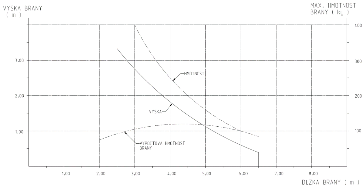
VZTAH VYSKY A HMOTNOSTI PLNEJ BRANY OD JEJ DLZKY
